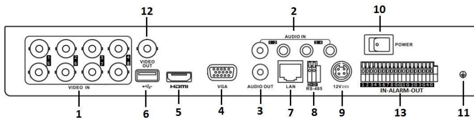
Obrázek 1–8–2 Popis konektorů zadního panelu verze 2
