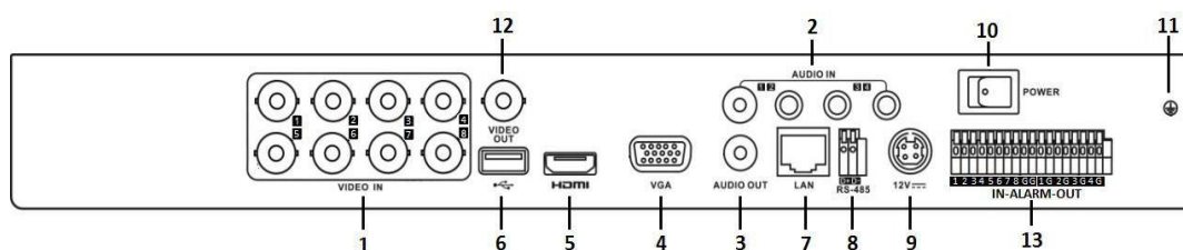
Obrázek 1–8–4 Popis konektorů zadního panelu verze 5
