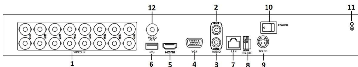
Obrázek 1–8–5 Popis konektorů zadního panelu verze 6
