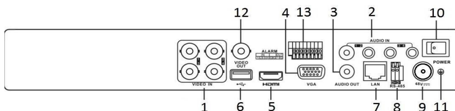
Obrázek 1–8–2 Popis konektorů zadního panelu verze 3
