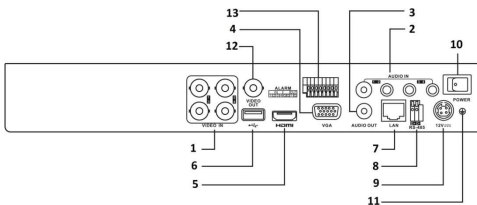
Obrázek 1–8–3 Popis konektorů zadního panelu verze 4
