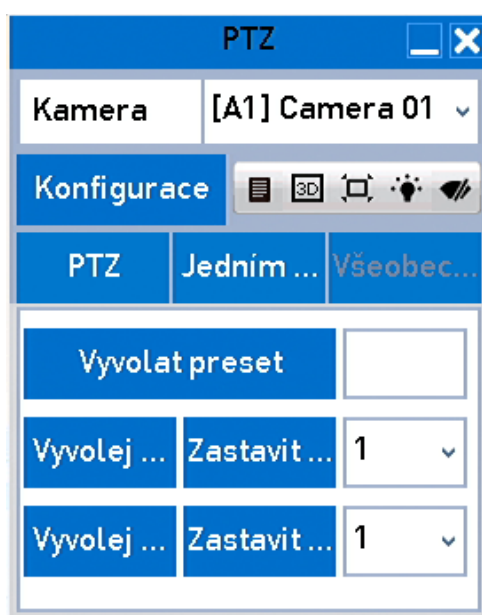
Obrázek 4–8 Panel PTZ
