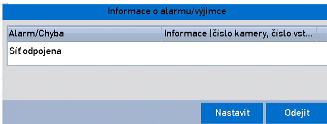
Obrázek 8–13 Podrobná událost
