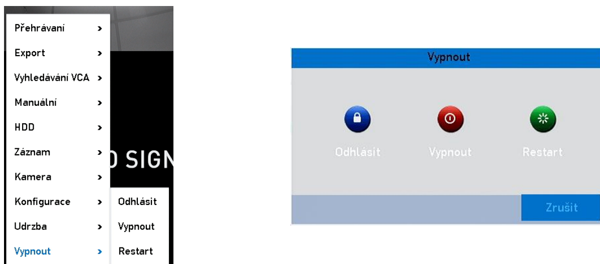
Obrázek 2–18 Odhlášení
