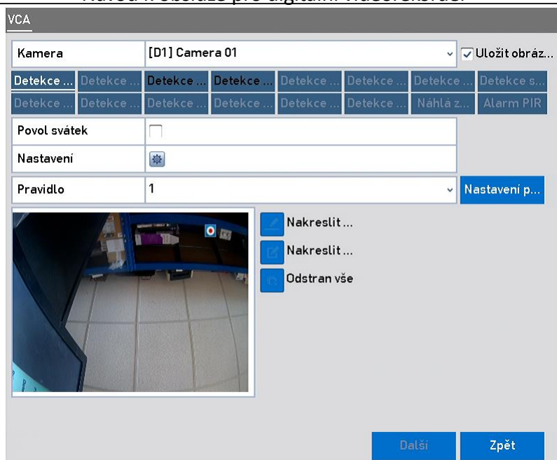
Obrázek 9–1 Detekce obličeje
