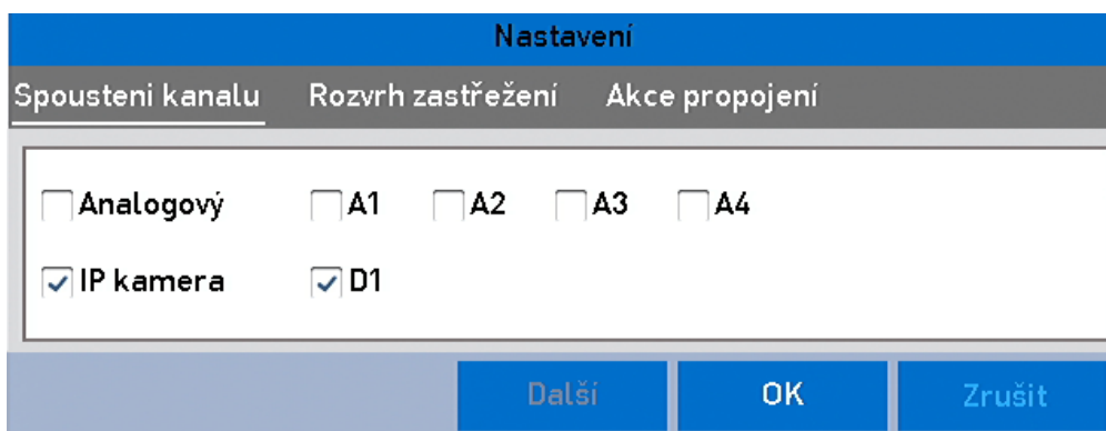
Obrázek 9–2 Propojení PTZ
