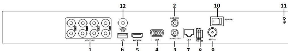
Obrázek 1–8–6 Popis konektorů zadního panelu verze 7
