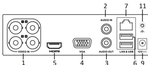
Obrázek 1–8–1 Popis konektorů zadního panelu verze 1
