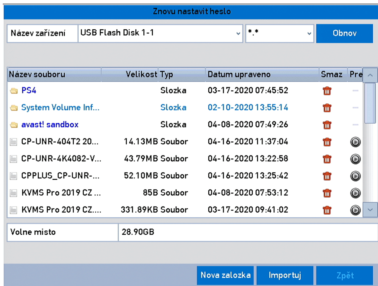
Obrázek 2–19 Importování GUID
