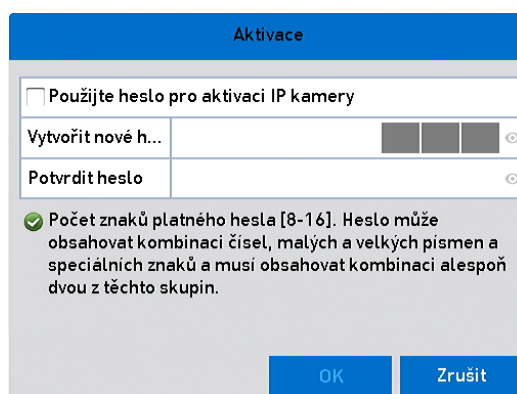
Obrázek 2–22 Aktivace kamery
