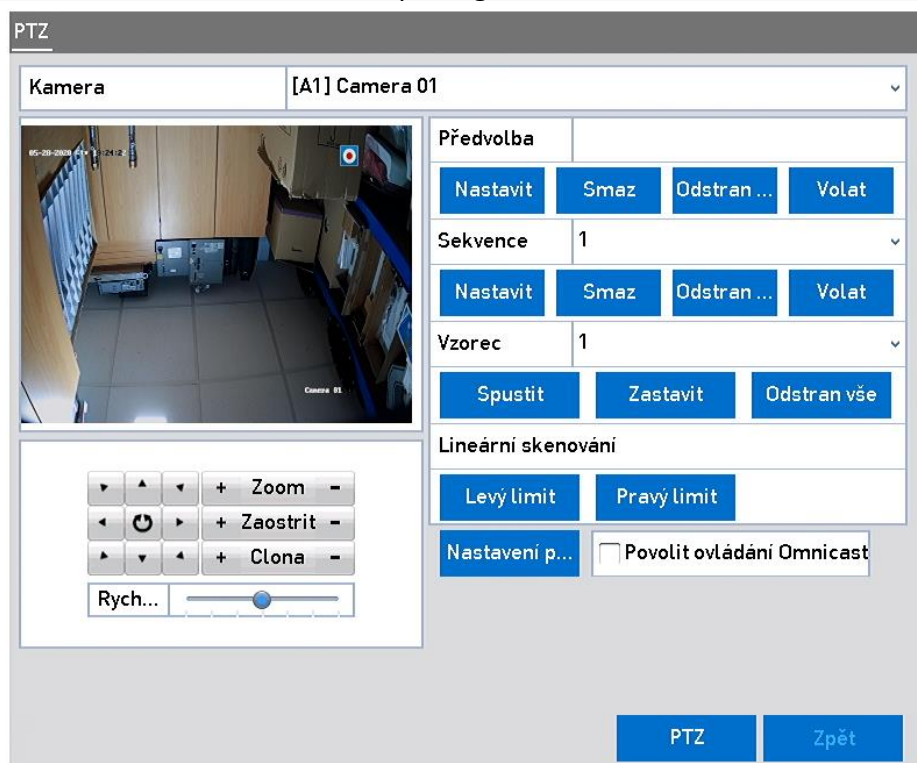
Obrázek 4–6 Nastavení PTZ
