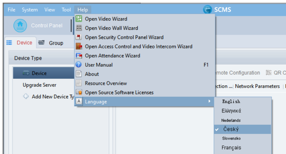
Obrázek 11-44 – Nastavení jazyka
