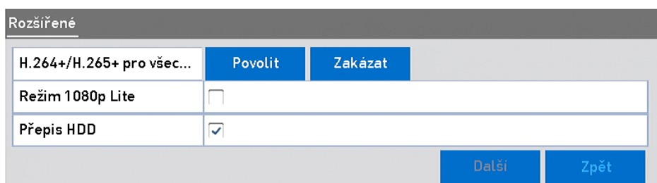
Obrázek 5–32 Rozšířené rozhraní
