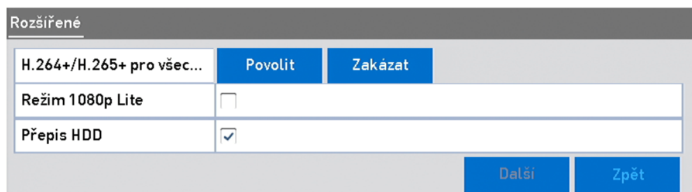
Obrázek 5–29 Pokročilá nastavení
