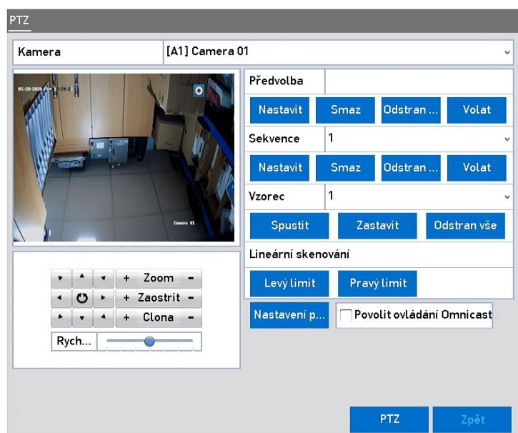
Obrázek 4–11 Nastavení PTZ
