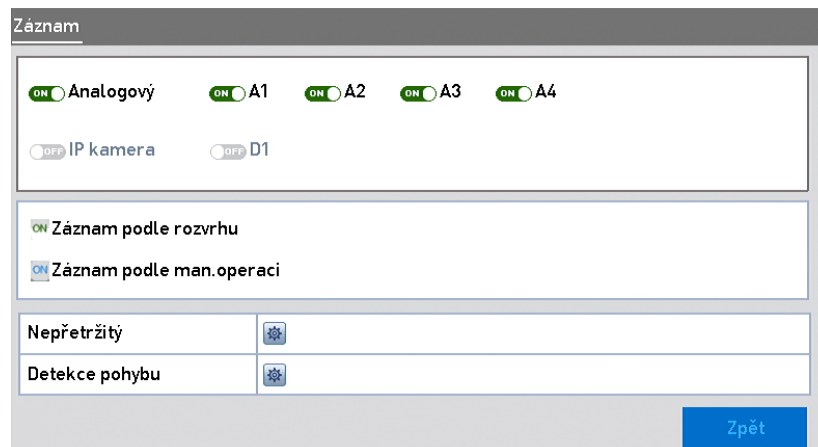
Obrázek 5–19 Ruční nahrávání
