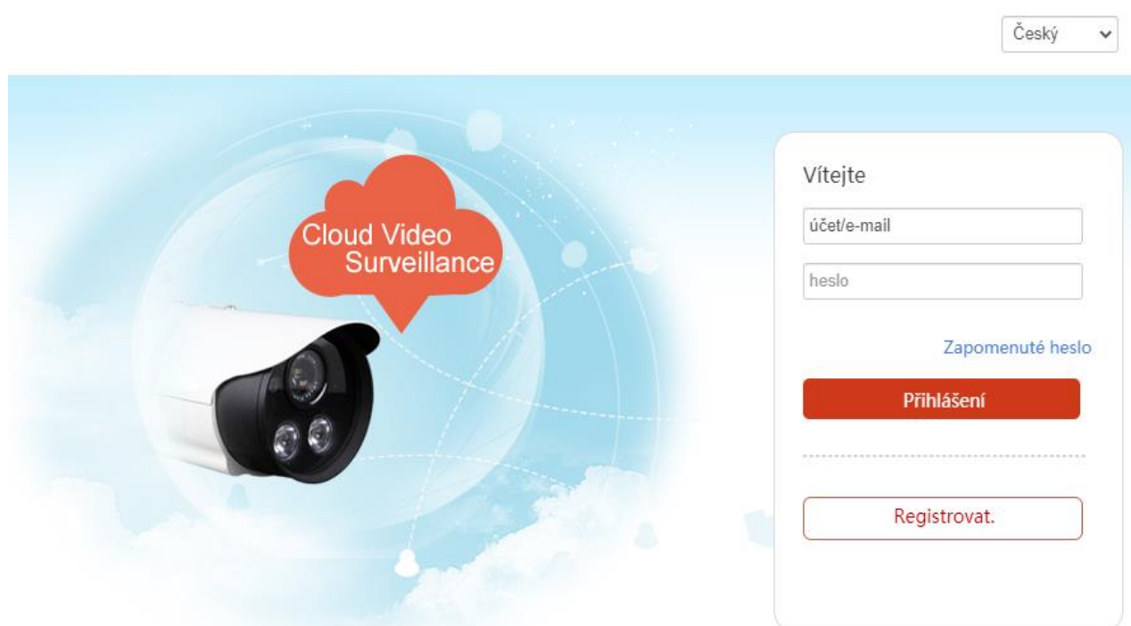
Obrázek 11-31 – Webová stránka
