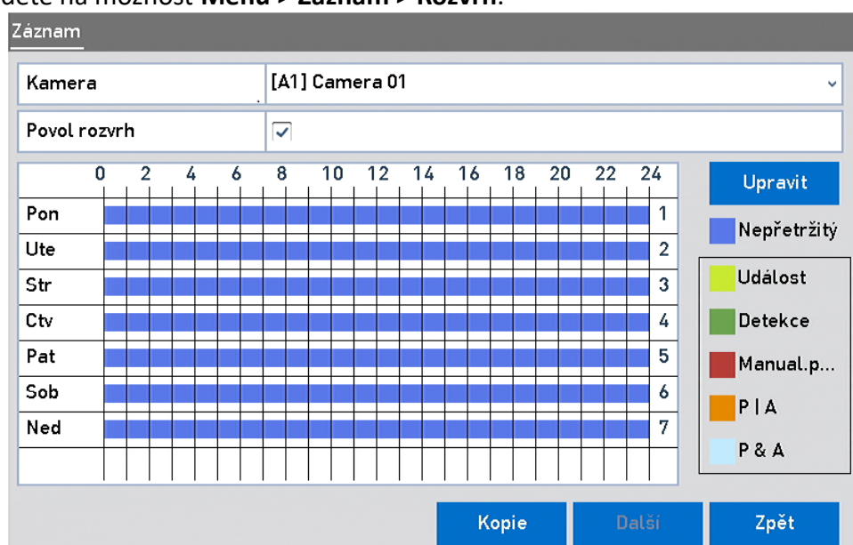
Obrázek 5–10 Plán nahrávání
