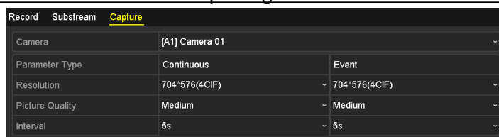
Obrázek 5–9 Nastavení snímků
