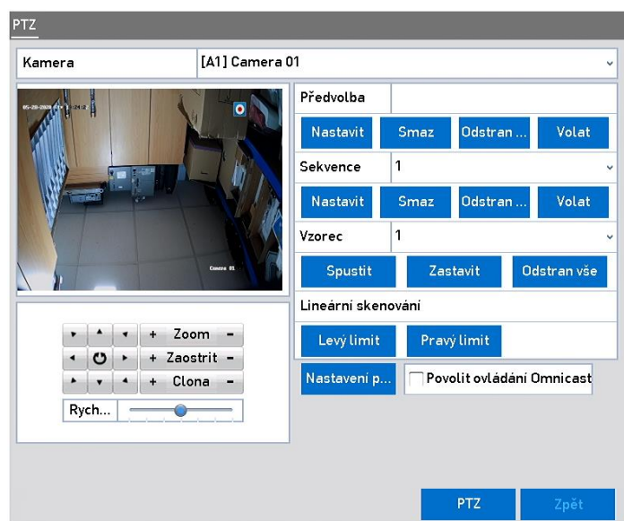
Obrázek 4–4 Nastavení PTZ
