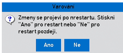
Obrázek 5–33 Upozornění
