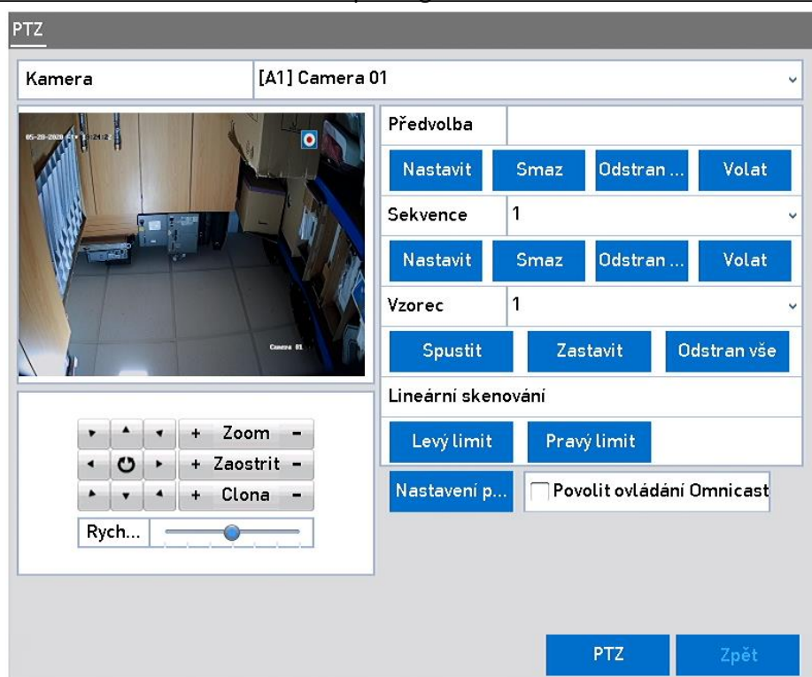
Obrázek 4–9 Nastavení PTZ
