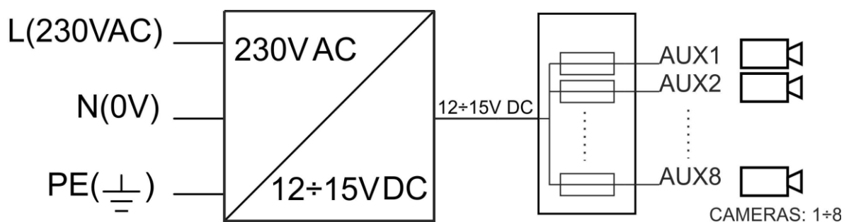
Obr. 1. Blokové schéma napájecího zdroje.
