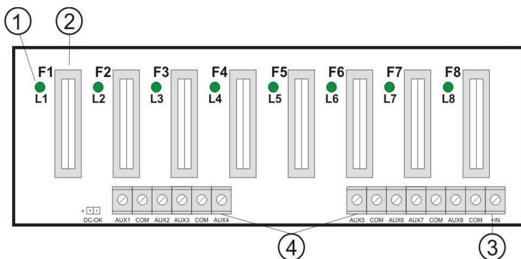
Obr. 2. Náhled na pcb jedné desky (ze dvou).
