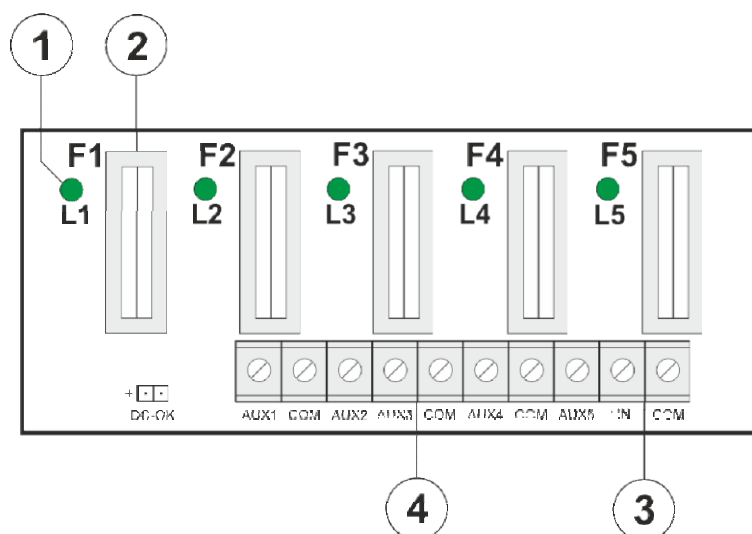
Obr. 2. Náhled na pcb jedné desky (ze dvou).
